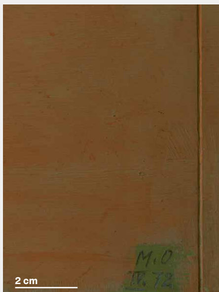
Abb. 4.9 Detail UV-Fluoreszenz-Signatur.
